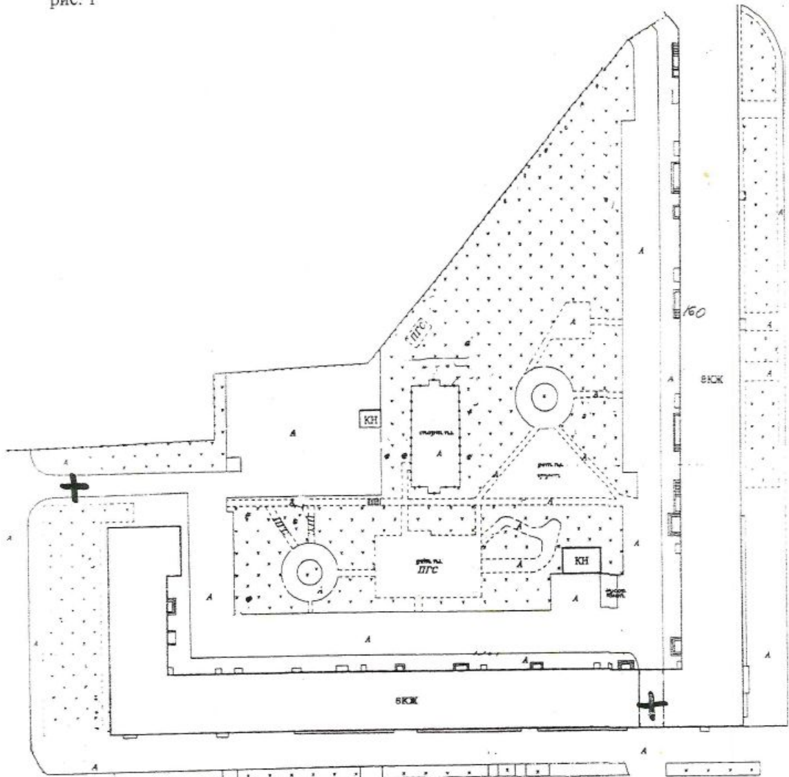
Рис. 1. Схема размещения ограждающих устройств
